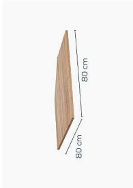
Eckverbindungsplatte 1708 mit Metall-Montageschrauben, optional mit Stützfuß [1702] ABS-Kanten, optional mit Stützfuß [1702] oder höhenverstellbarem Stützfuß [1705]
