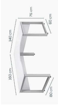
Schreibtisch 1712 (160 x 140 cm) Winkelkombination mit Metallgestell linker Schenkel 160 x 80 cm rechter Schenkel 140 x 60 cm
