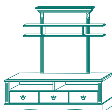
Kombination 4 142x185x56cm
